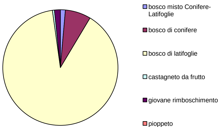
Grafico C.2 – Analisi tipologie forestali per famiglie
